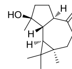
Spathulenol
